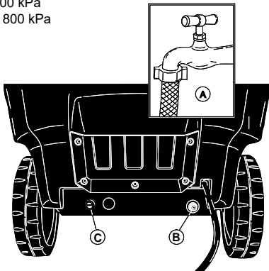
Tilkobling til vannettet.
